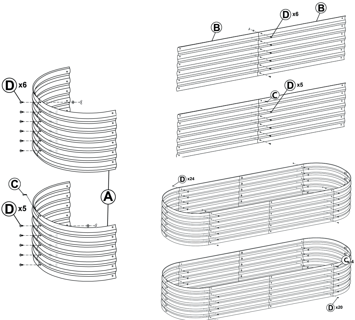
Ausführung niedrig
